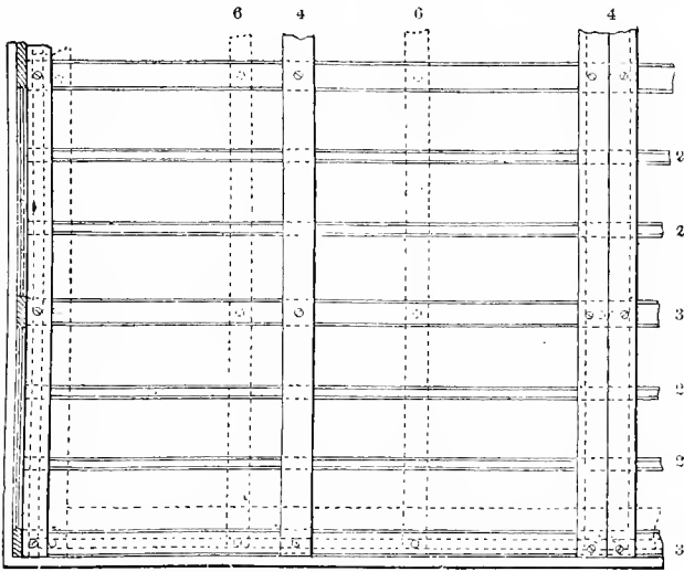
Fig. 2356. Plan.
